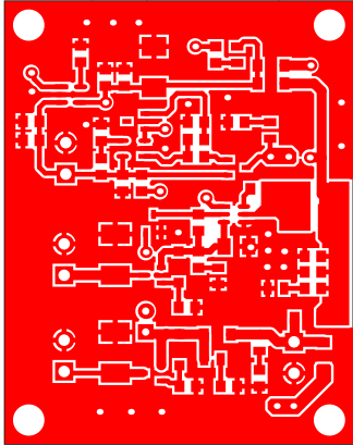
Top Layer (Scale 1:1) [Top]
